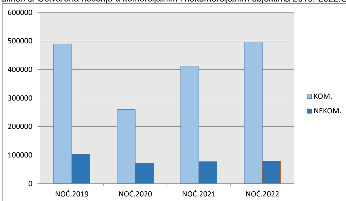
Grafikon 3. Ostvarena noćenja u komercijalnim i nekomercijalnim objektima 2019.-2022.G.
